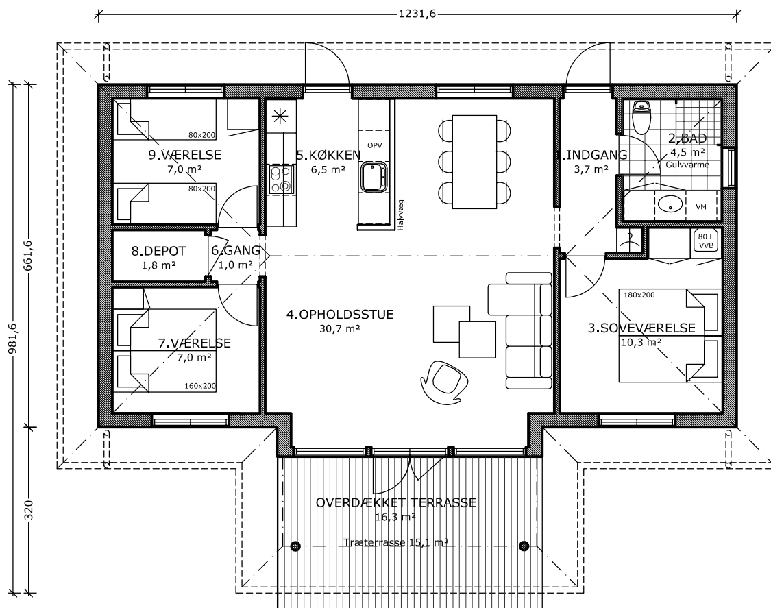
Stueplan 1:100
