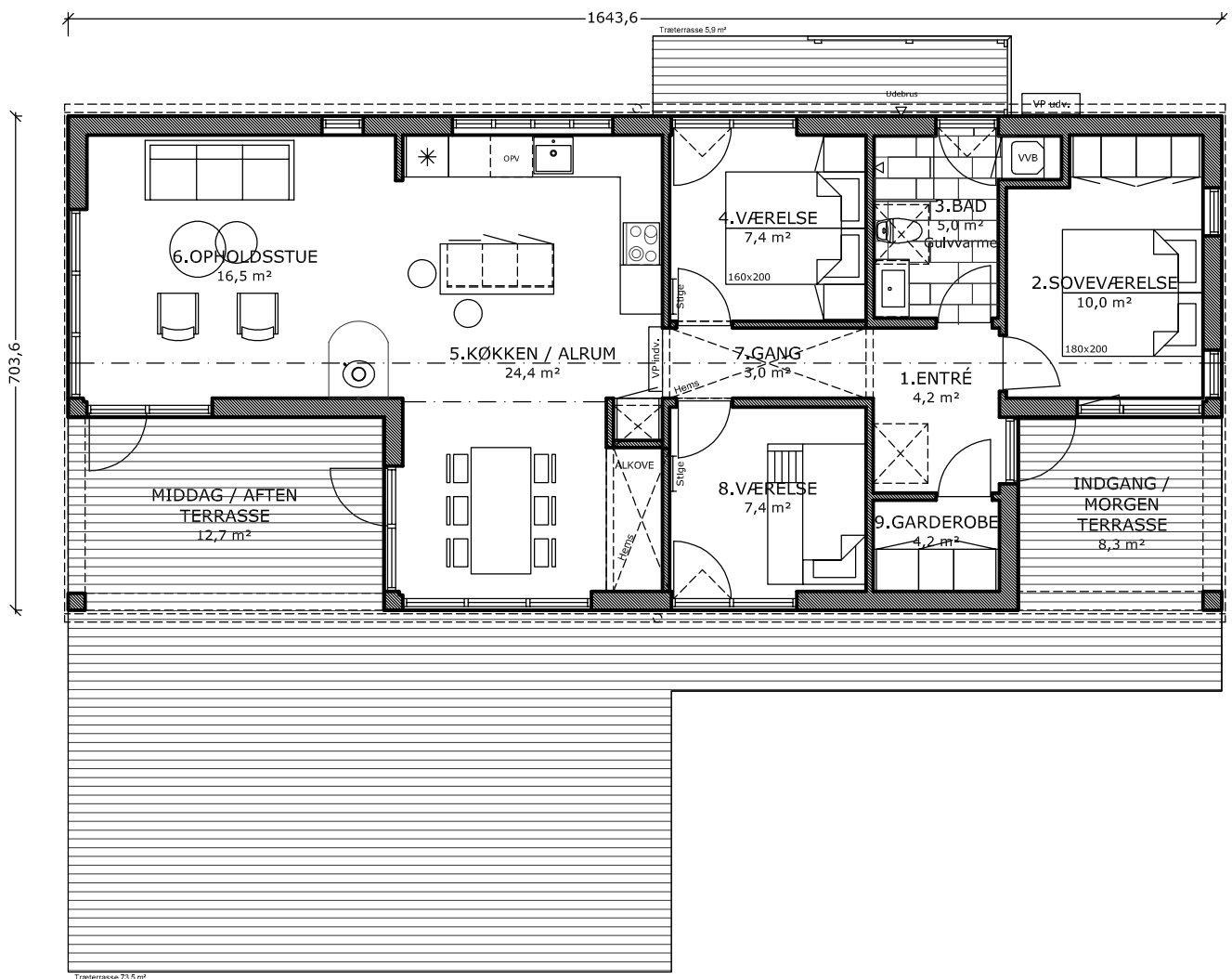
Stueplan 1:100
