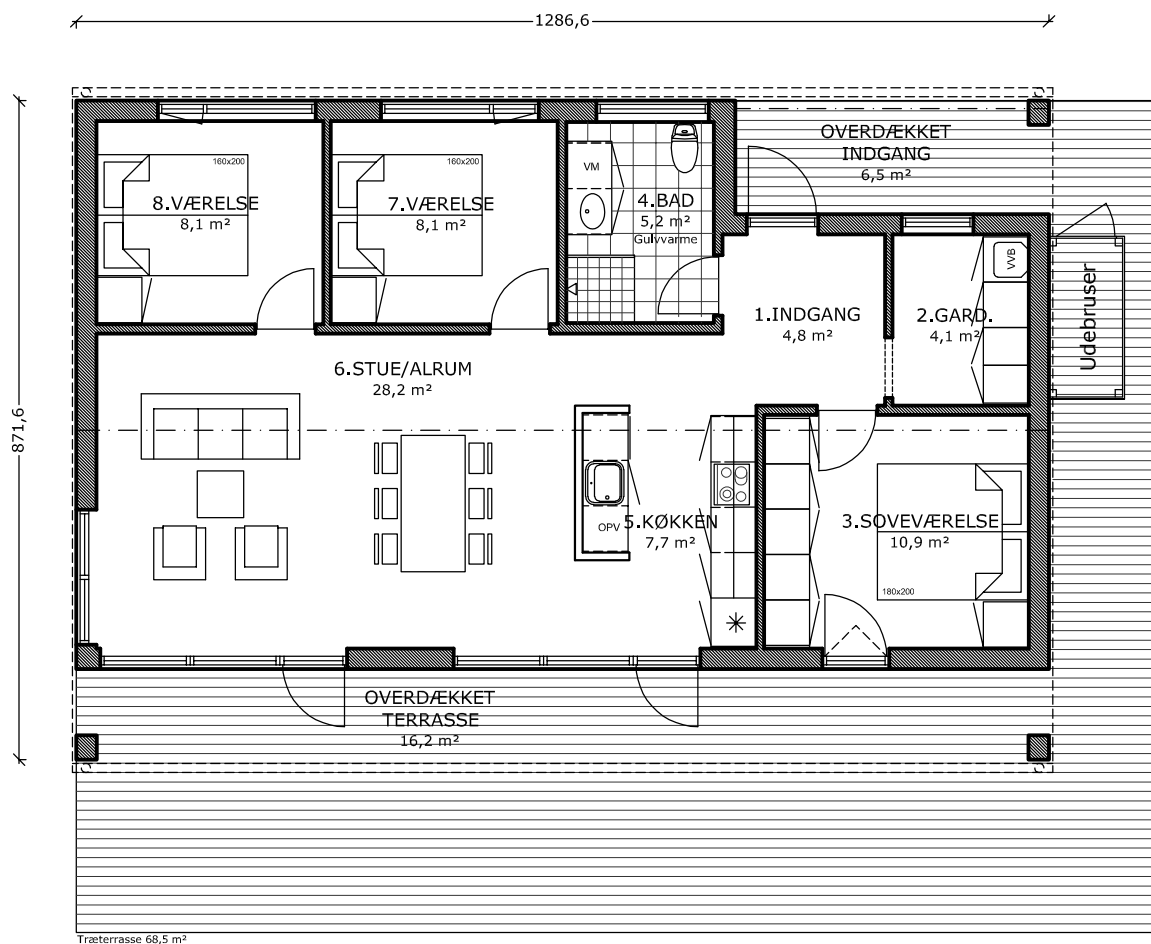
Stueplan 1:100
