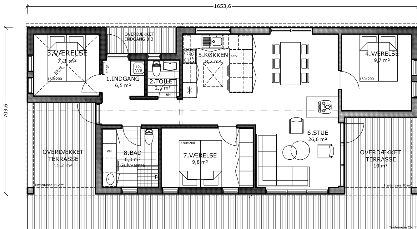
Stueplan 1:100
